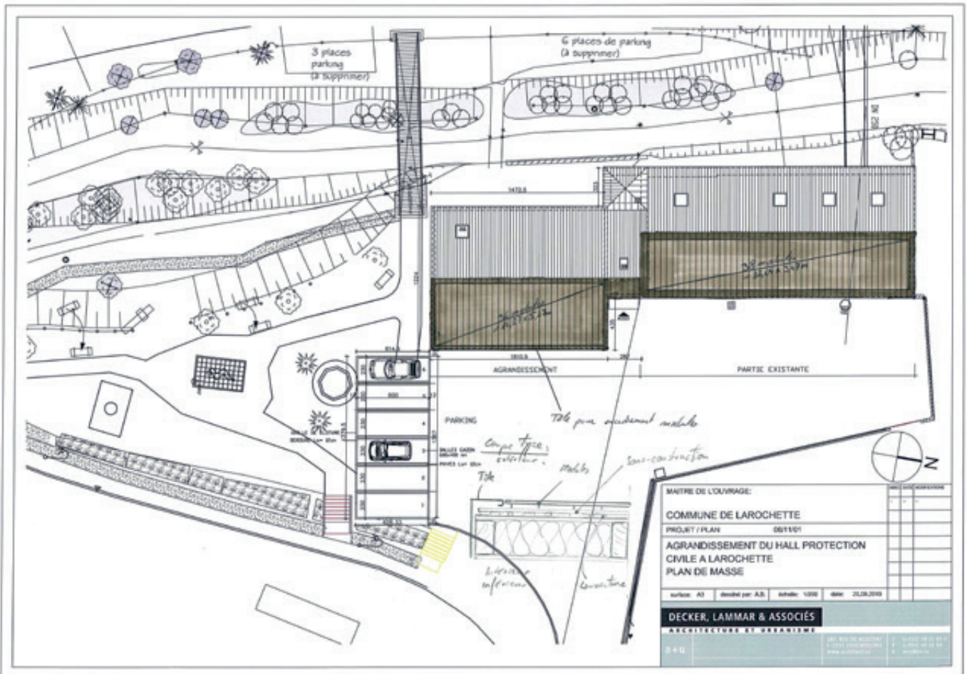
Surface projetée pour installation photovoltaïque Geplante Fläche für die Photovoltaik-Anlage
